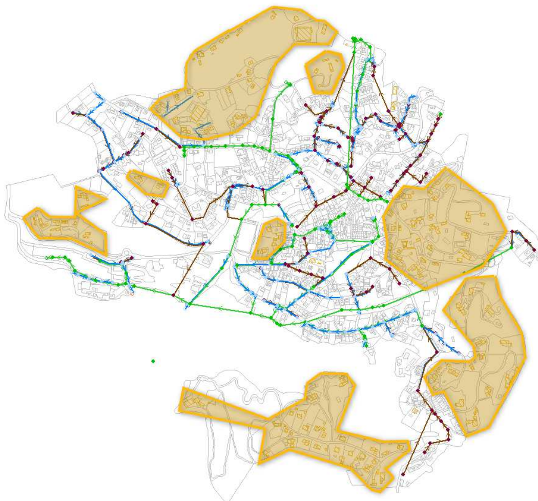
Figura 12. Zones on es sospita de l'existència de fosses sèptiques.
