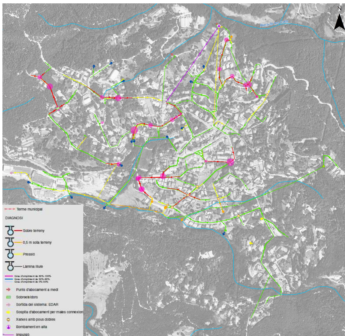
Figura 37. Funcionament de la xarxa pluvial i unitària per a una pluja de T=10 anys.
