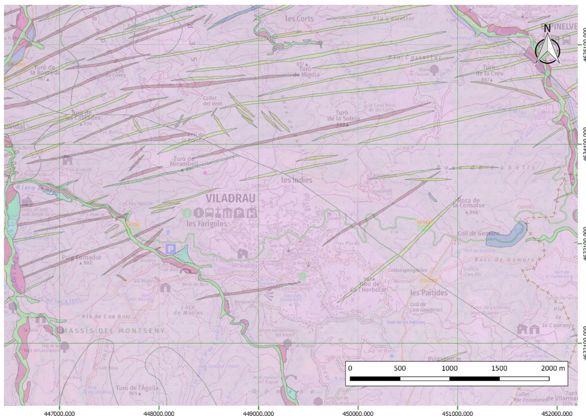
Figura 1. Mapa geològic de la zona (Geològic 1:25000 ICGC)
