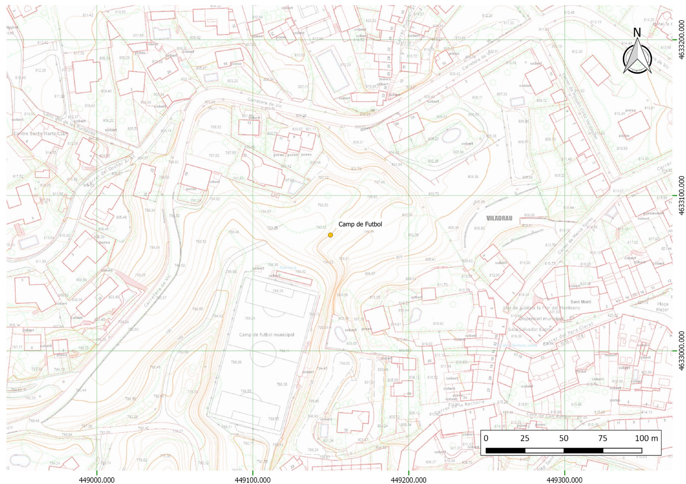
Figura A2 06. Proposta de prospecció al Camp de futbol
