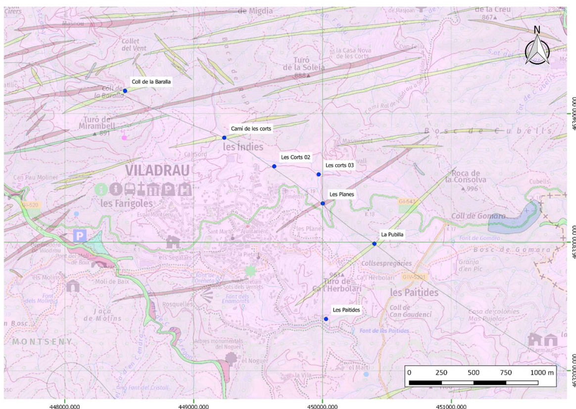
Figura 3. Localització de les propostes de prospecció tenint en compte els criteris geològics.
