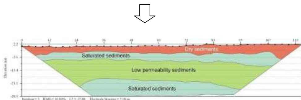
Interpretació de la pseudosecció geoelectrica 2D
